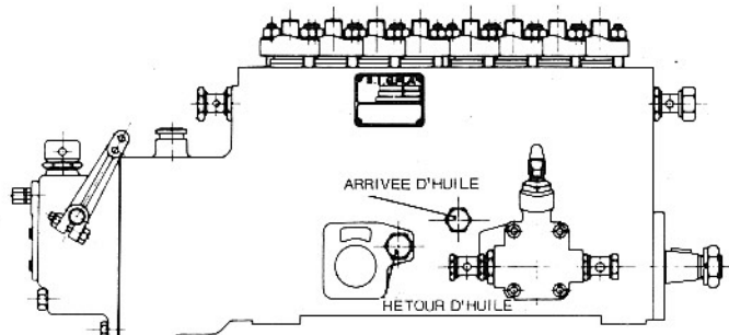
PLAN DE LA POMPE D'INJECTION : réf. 672053 à l'indice : G
