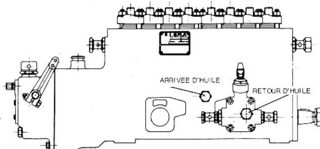
PLAN DE LA POMPE D'INJECTION : réf. 672053 à l'indice : H
